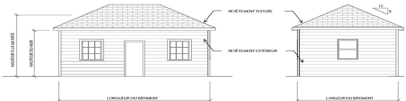
ÉLÉVATION AVANT
