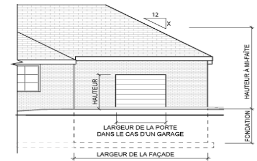
ÉLÉVATION AVANT
