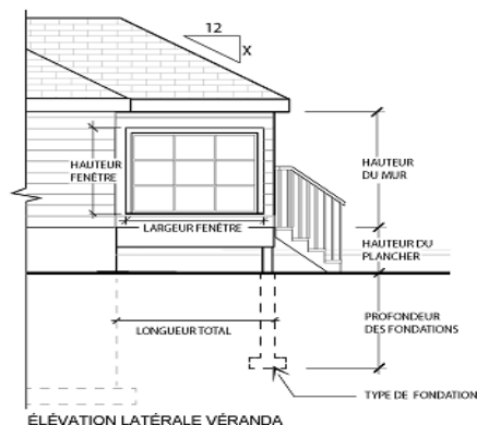
ÉLÉVATION LATÉRALE VÉRANDA
