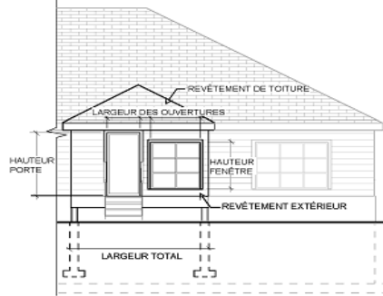
ÉLÉVATION ARRIÈRE VÉRANDA
