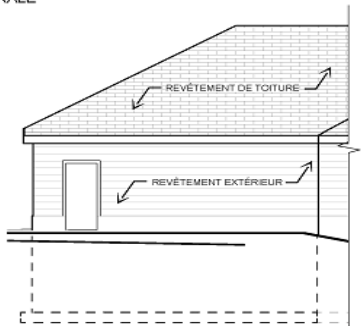
ÉLÉVATION ARRIÈRE GARAGE
