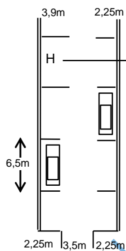
STATIONNEMENT PARALLÈLE
