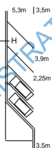
STATIONNEMENT À 30°
