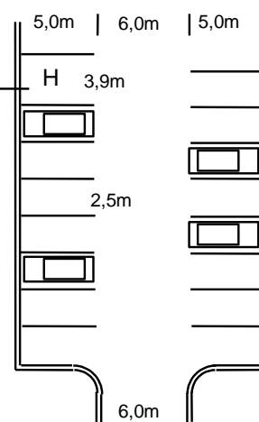
STATIONNEMENT À 30°
