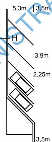
STATIONNEMENT À 30°
