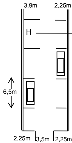
STATIONNEMENT PARALLÈLE
